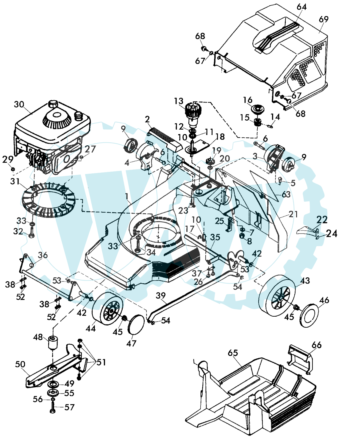
40 BK V12 - Art.78570 ab Baujahr 1990
